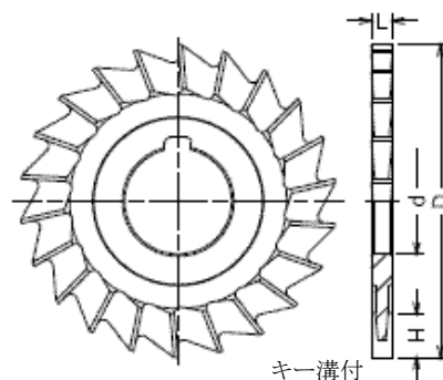
キー溝付
