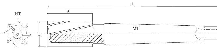
MT1シャンク
