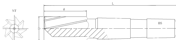
BS5シャンク
