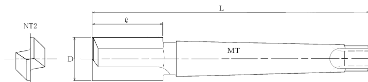
MT1シャンク
