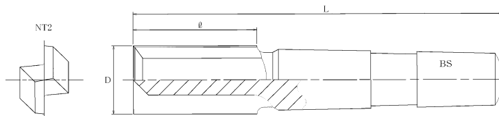
BS5シャンク
